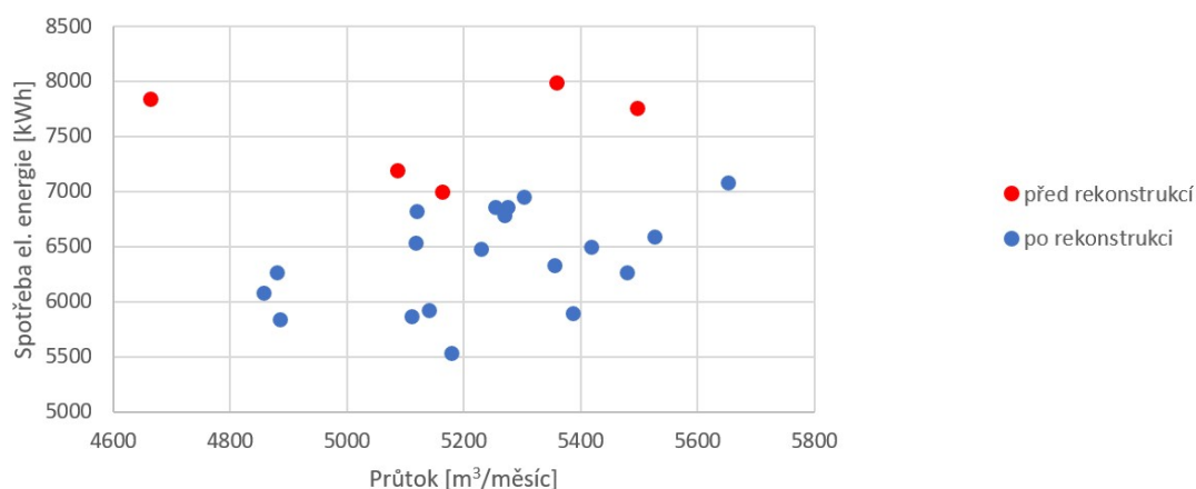
ČOV Kupařovice - efektivita provozu
